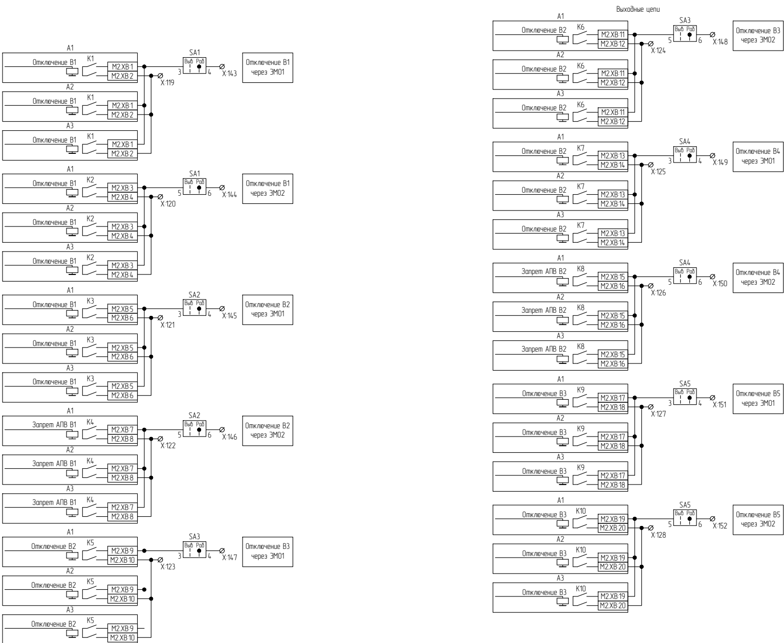
Рисунок Г.6 – Схема электрическая принципиальная (часть 6)
